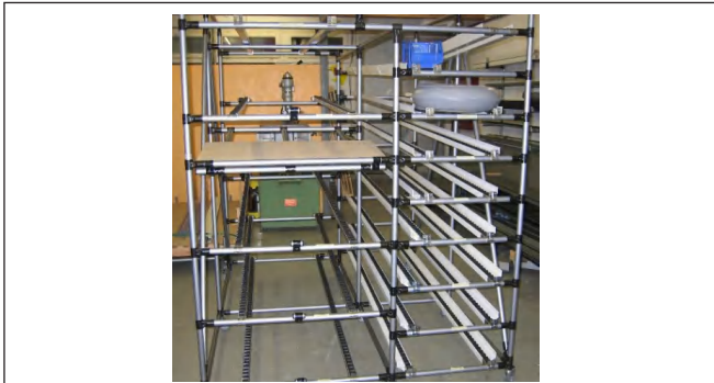
017 打包台货架
